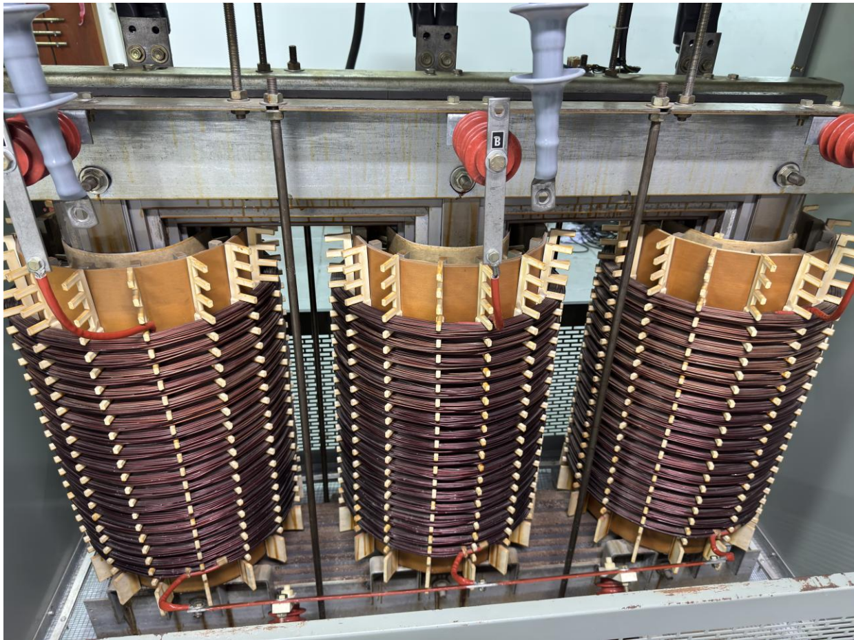
VII.2.c - Bên trong phía cao áp MBA kích từ TE1
