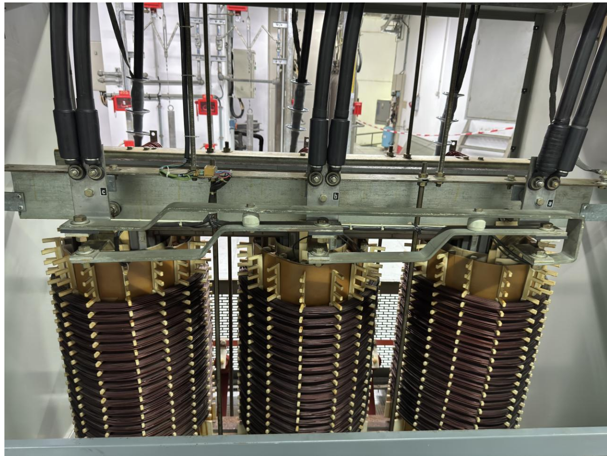
VII.2.d - Bên trong phía hạ áp MBA kích từ TE1
